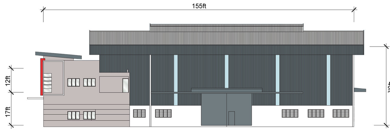
RIGHT ELEVATION
